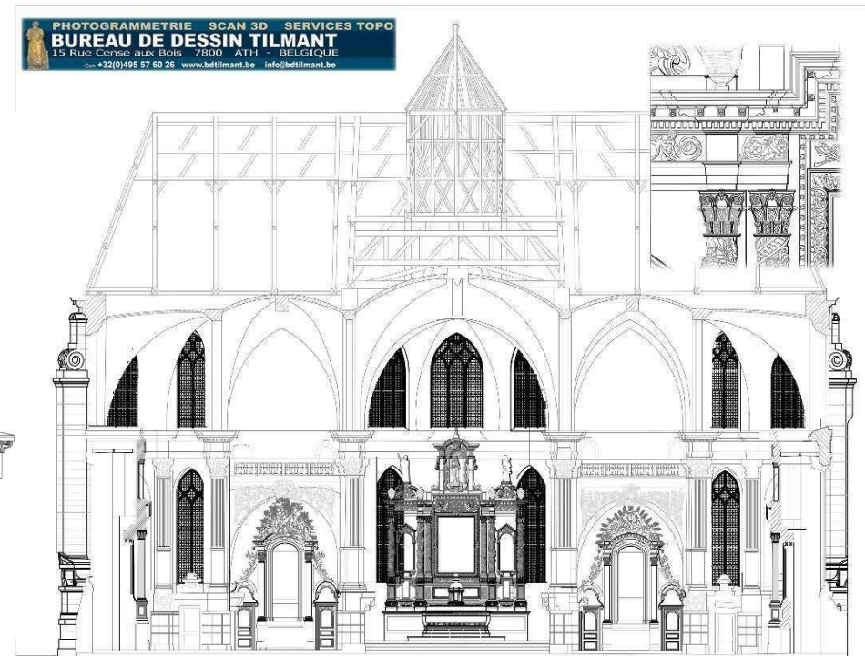
Coupe - Chapelle Corneille - Rouen
